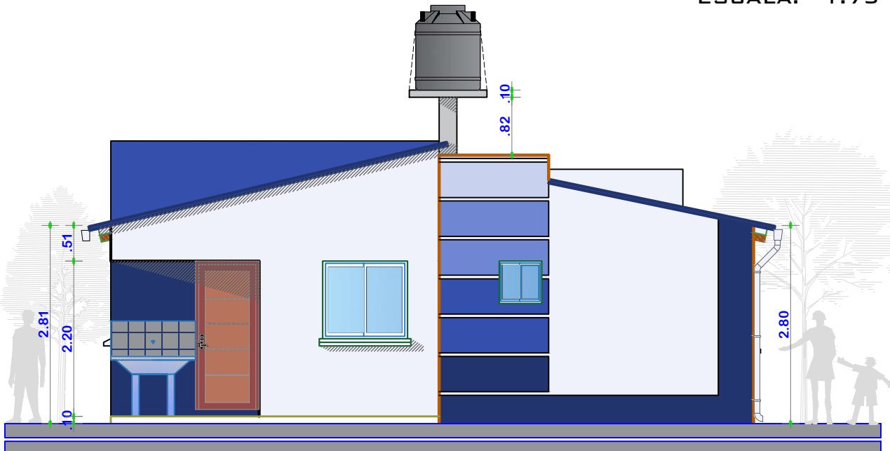
ELEVACION POSTERIOR
