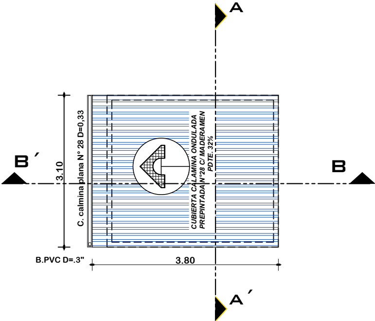
PLANO ESTRUCTURAL DE CUBIERTAS ESCALA: 1:75
