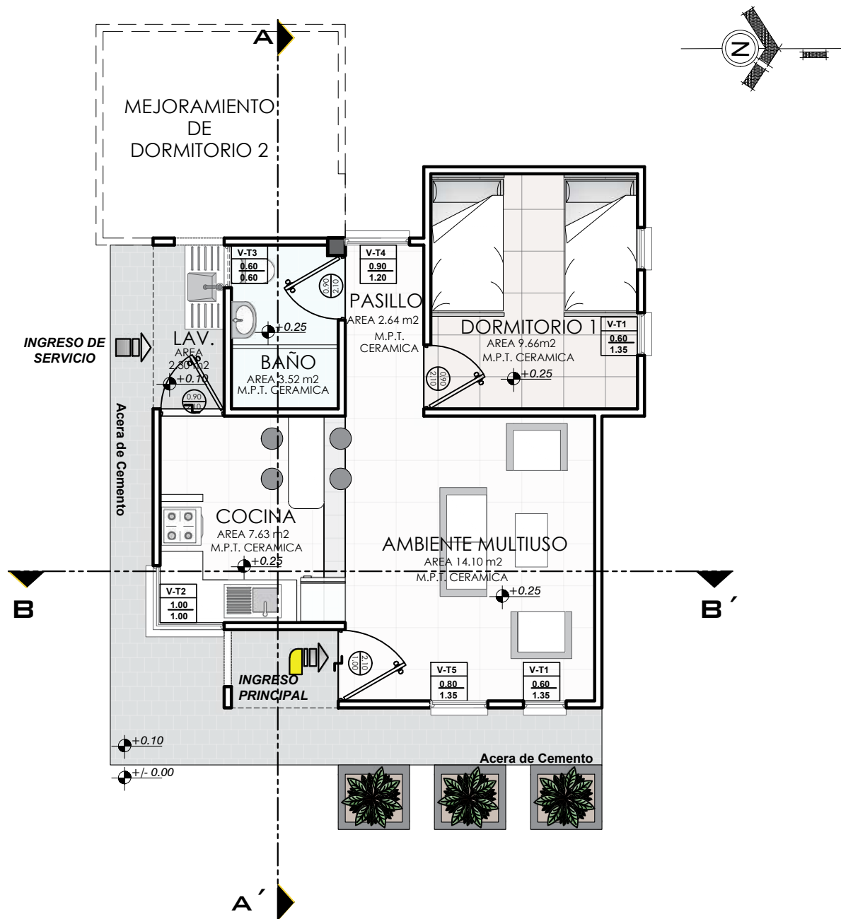
PLANTA AMOBLADA ESCALA: 1:75
