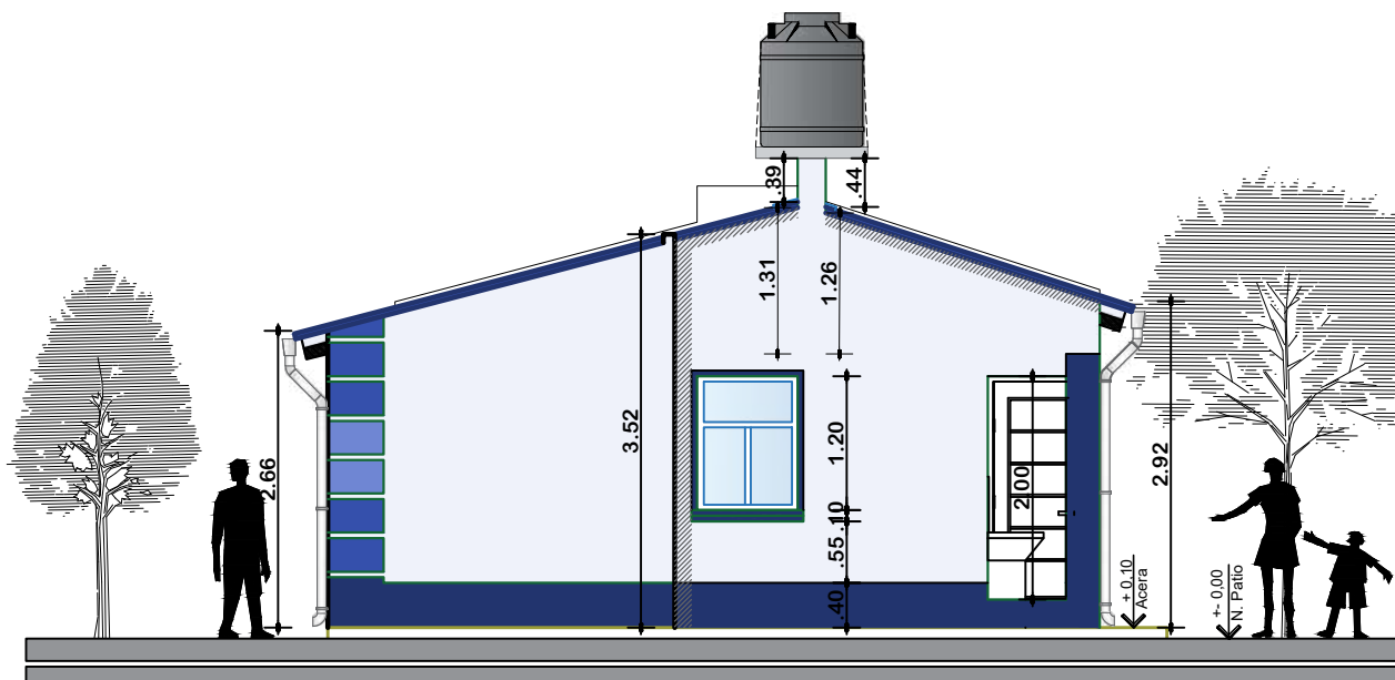
ELEVACION POSTERIOR ESCALA: 1:75
