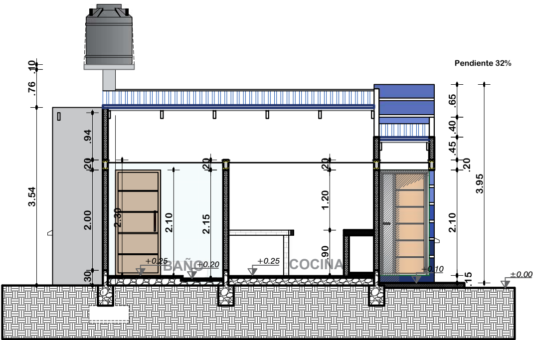
CORTE A-A' ESCALA: 1:75
