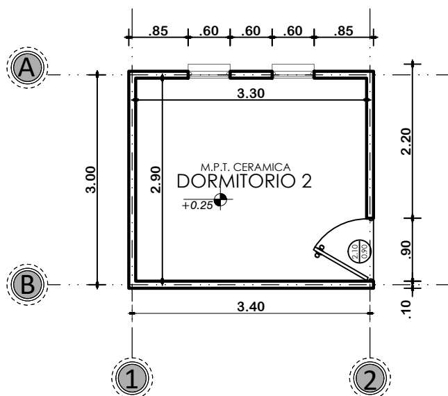
PLANTA ACOTADA ESCALA: 1:75
