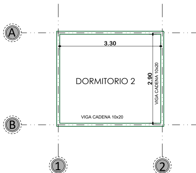
PLANO DE VIGA DE HºAº ESCALA: 1:75
