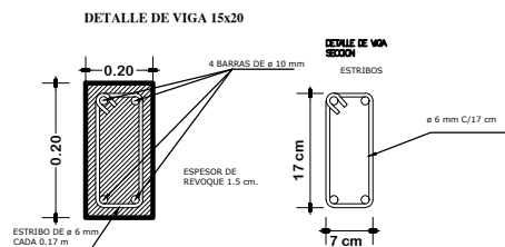
PLANTA DE VIGA DE H°A° ESCALA: 1:75
