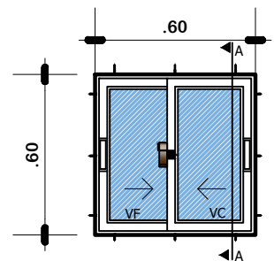
ELEVACION
