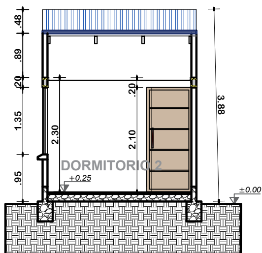
CORTE A-A' ESCALA: 1:75
