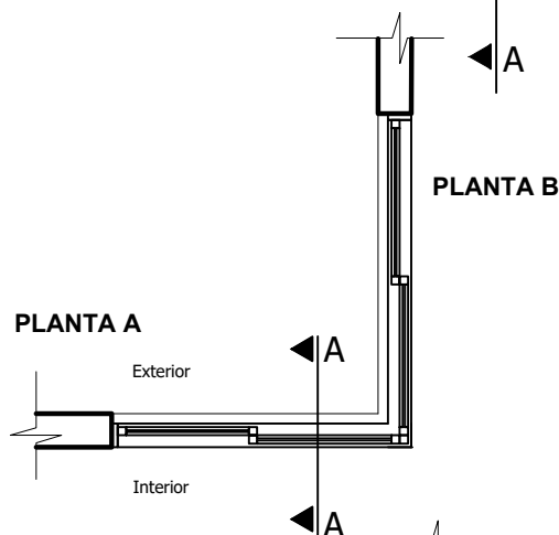
VENTANA TIPO 2 DETALLE VENTANA DE ALUMINIO 1,00 x 1,00 ESC: 1:25
