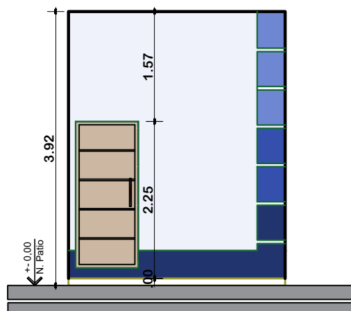
ELEVACION LATERAL ESCALA: 1:75
