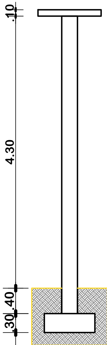
DETALLE COLUMNA DE HºAº Y ZAPATA DE HºAº ESCALA: 1:50
