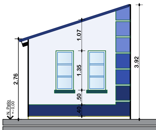
ELEVACION FRONTAL ESCALA: 1:75
