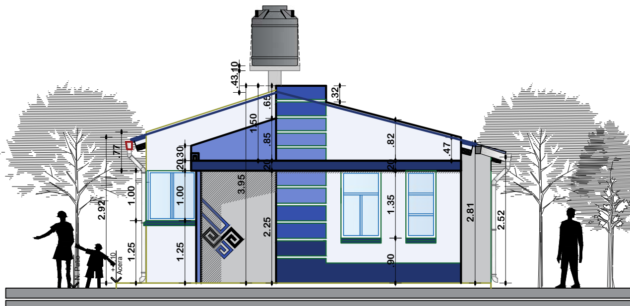
ELEVACION FRONTAL ESCALA: 1:75
