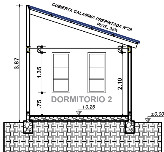
CORTE B-B' ESCALA: 1:75
