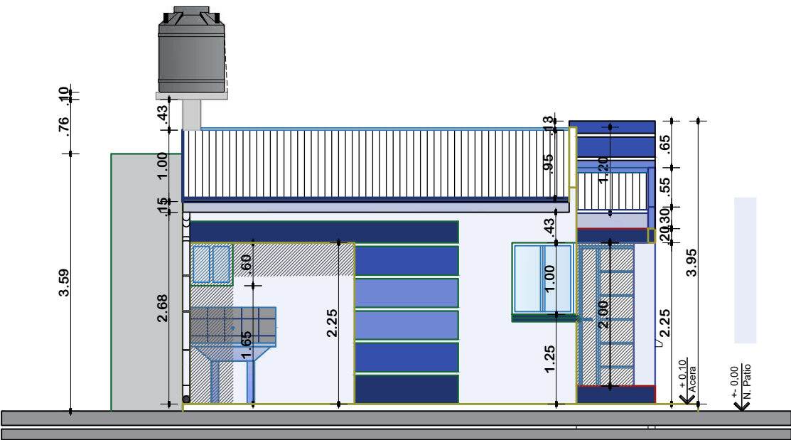
ELEVACION LATERAL DERECHO ESCALA: 1:75
