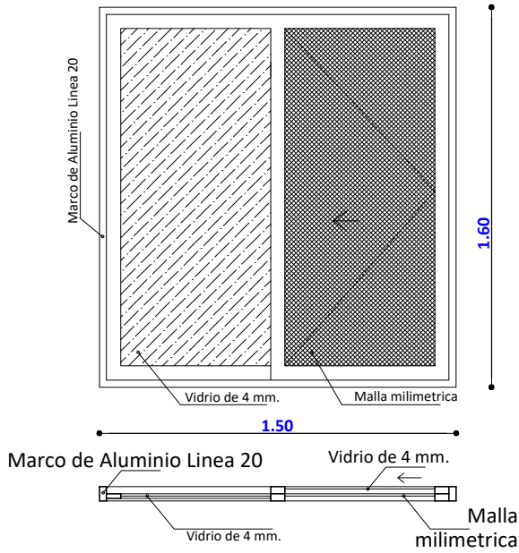
V-1 Ventana Tipo 1 1,50 1,60
