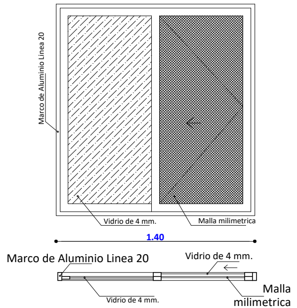
V-2 Ventana Tipo 2 1,40 1,60
