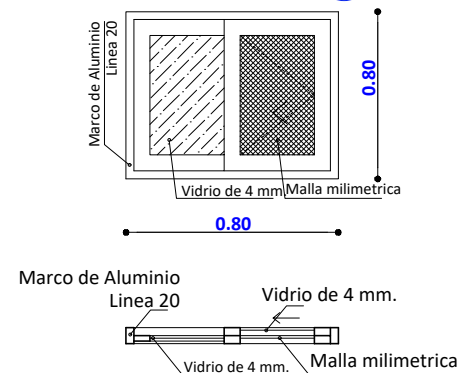
V-3 Ventana Tipo 3 0,80 0,80
