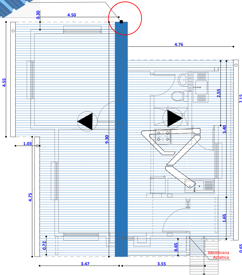
PLANO DE CUBIERTA ESC. 1:75
