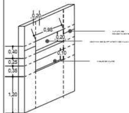
MURO DE BAÑO
