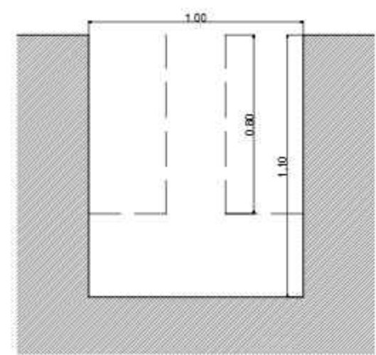
EXCAVACION DE ZAPATA TIPO 1
