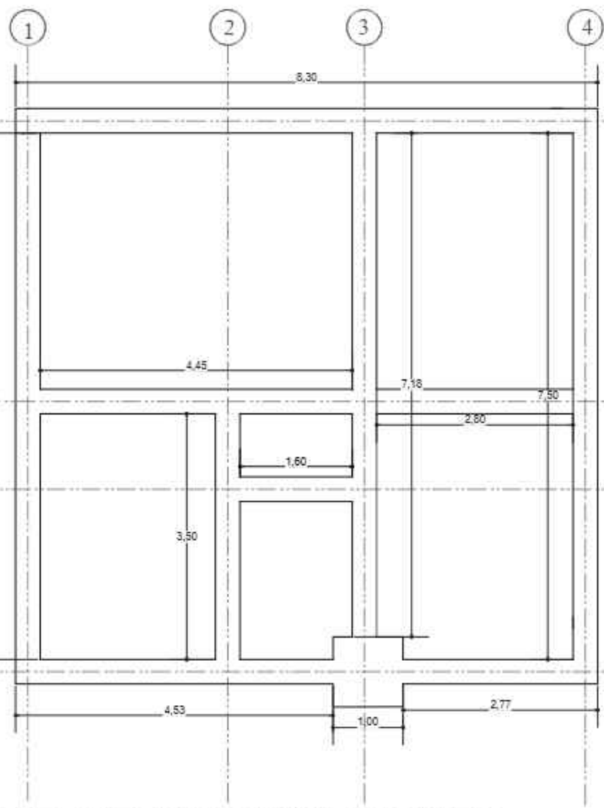
PLANO DE EXACAVACIONES ESCALA: 1:75
