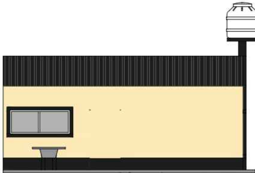
FACHADA LATERAL DERECHA ESCALA: 1:75
