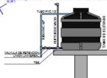
DETALLE DE TANQUE
