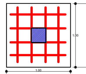
DETALLE DE COLUMNA DE TANQUE ELEVADO
