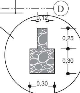
DETALLE DE CIMIENTO MURO BAÑO C 2-3
