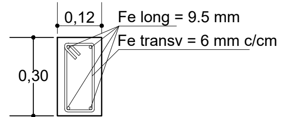
SECCIÓN DE VIGA CADENA DE H°A°
