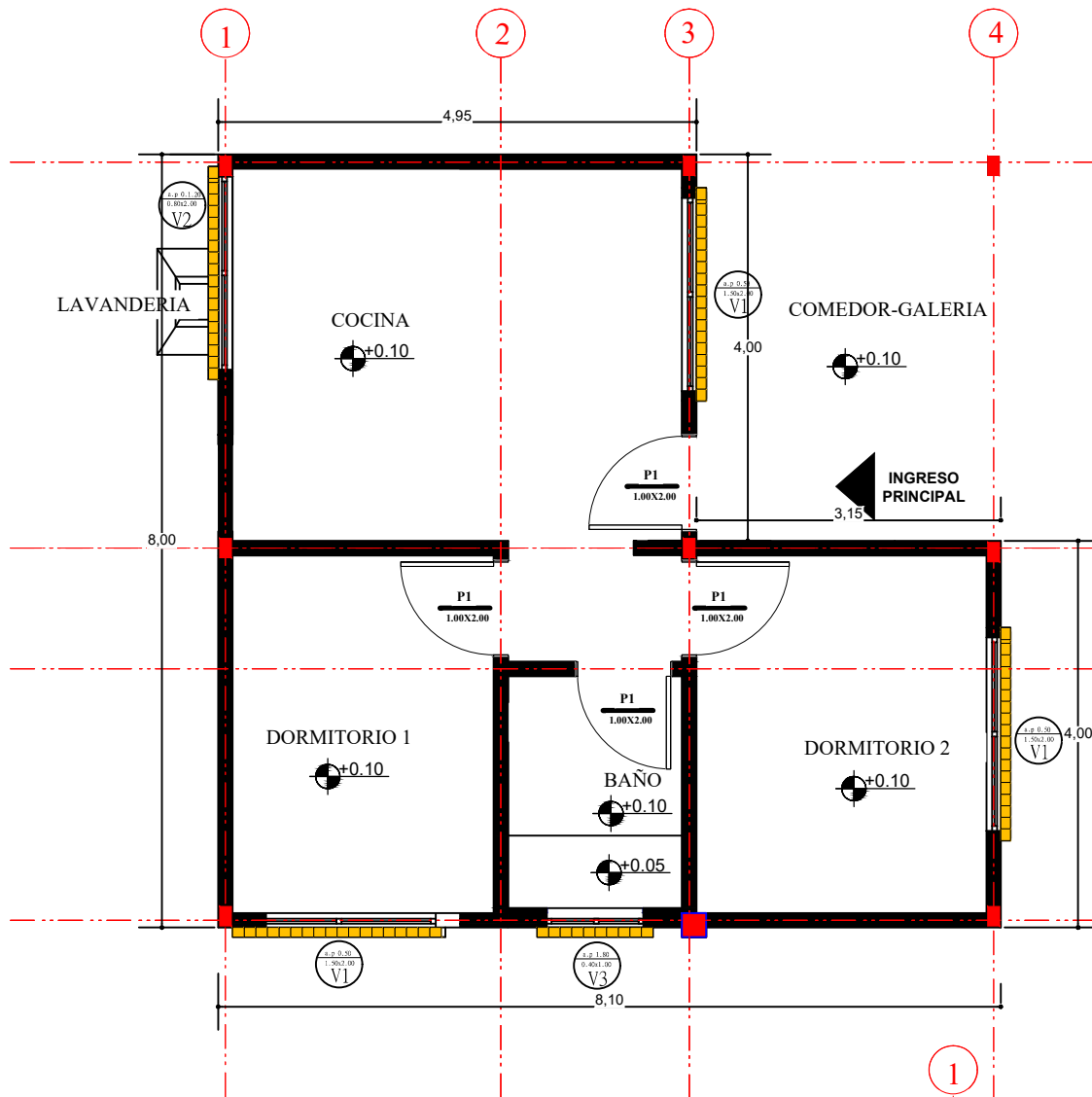
PLANO DE REVOQUE EXTERIOR ESCALA: 1:75
