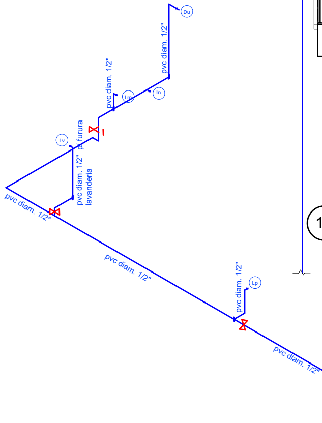
40 PLANO ESQUEMATICO ISOMETRICO - DE INSTALACION HIDRAULICA Scale: 1:100
