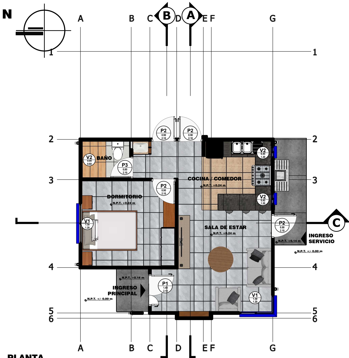
PLANTA ESC. 1:75
