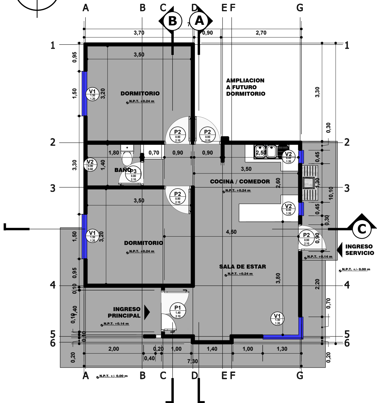
PLANTA ACOTADA ESC. 1:75
