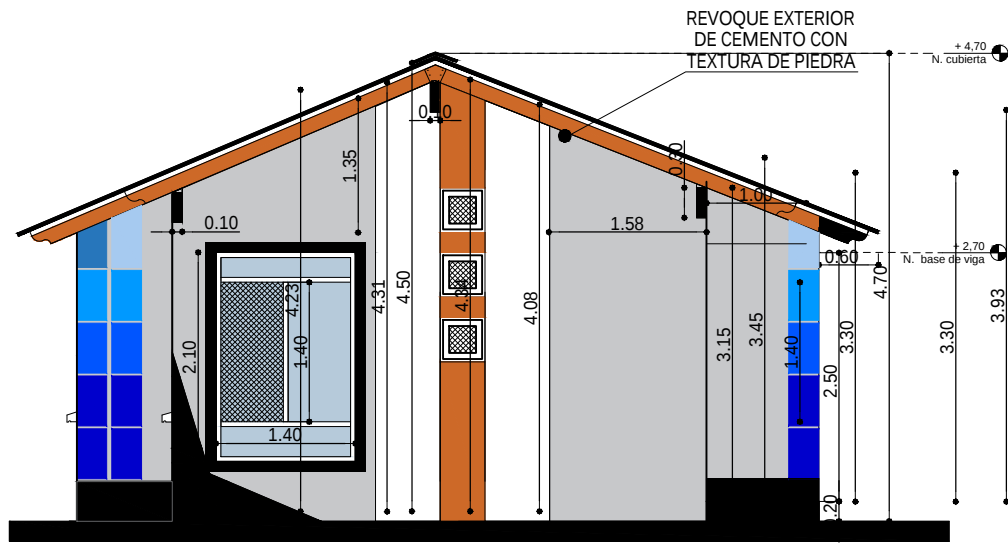
ELEVACION FRONTAL ESC. 1:75
