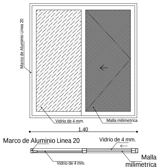
Ventana Tipo 2
