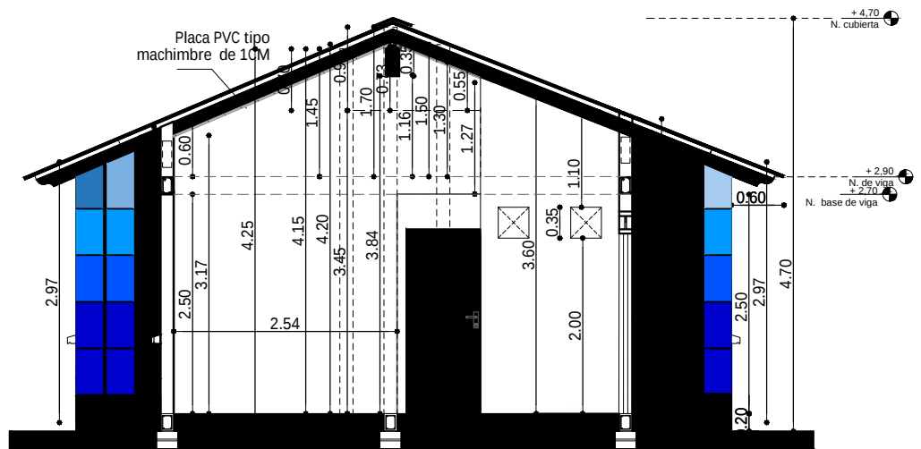
CORTE D-D"
