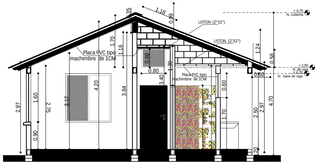
CORTE C-C"
