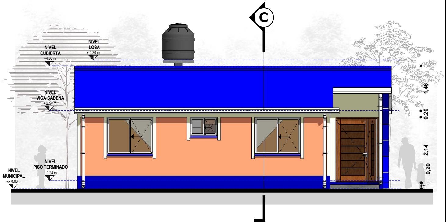
LATERAL ESC. 1:75
