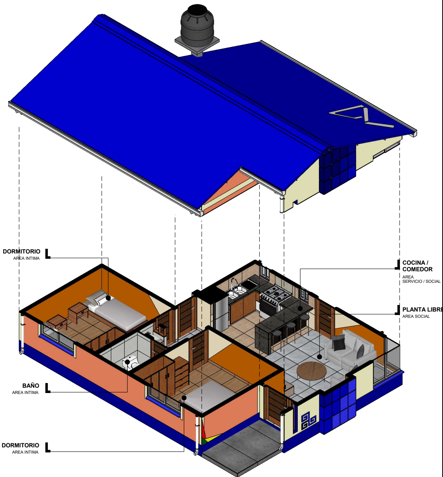
PLANTA ISOMETRICA ESC. 1:75
