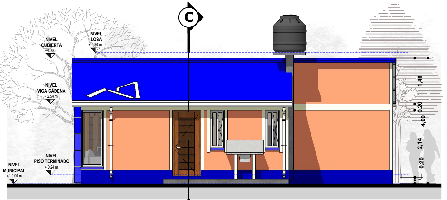
LATERAL ESC. 1:75
