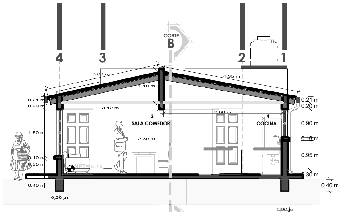
CORTE A-A
