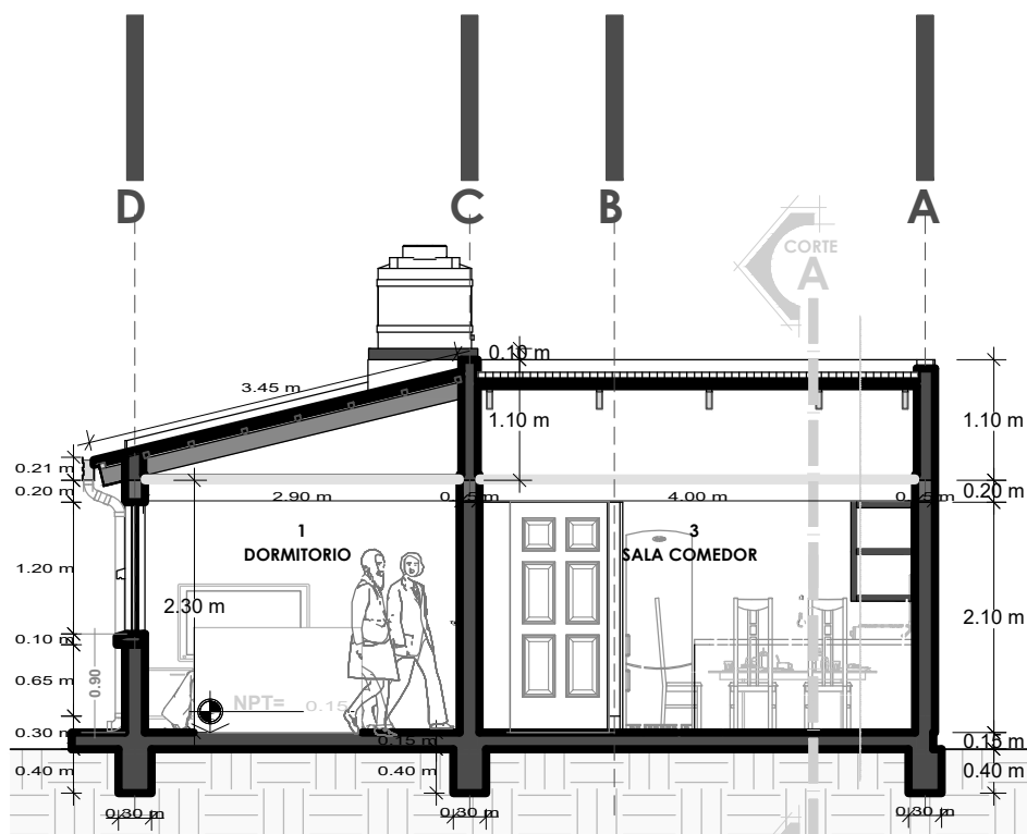
CORTE B-B
