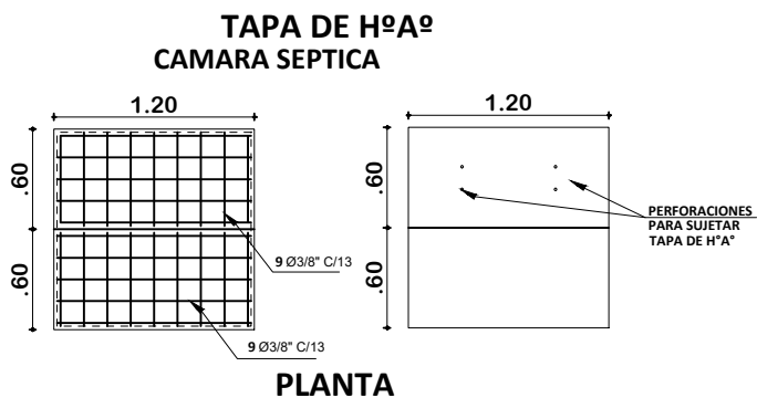
DETALLE CONSTRUCTIVOS POZO DE ABSORCION Y CAMARA SEPTICA ESCALA: 1:50
