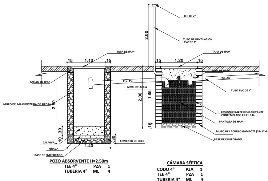
PLANO INSTALACION CAMARA Y POZO ABSORVENTE ESCALA: 1:75
