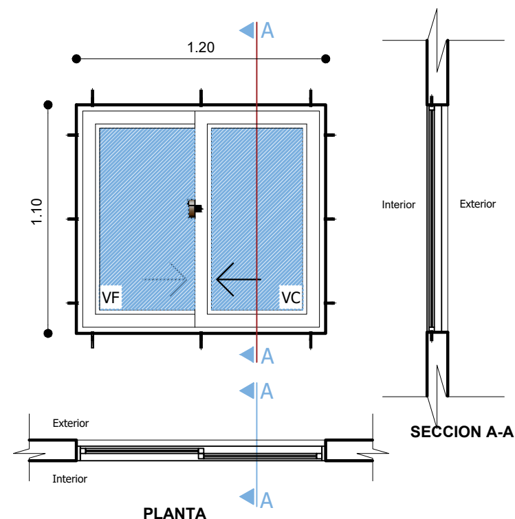
VENTANA TIPO 1 DETALLE VENTANA DE ALUMINIO 1.20 x 1.20 ESC.: 1:25
