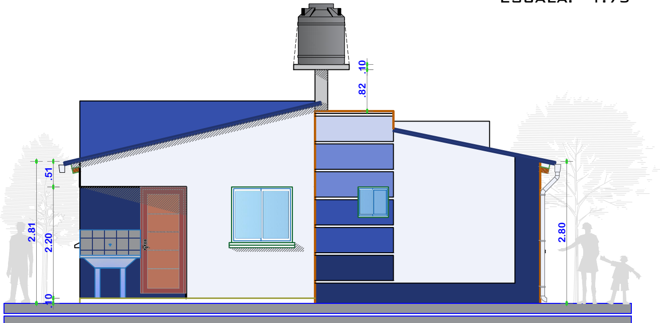
ELEVACION POSTERIOR
