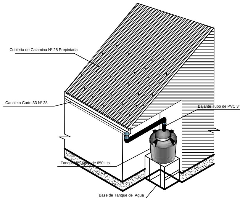
PERSPECTIVA COSECHA DE AGUA ESC. S/E
