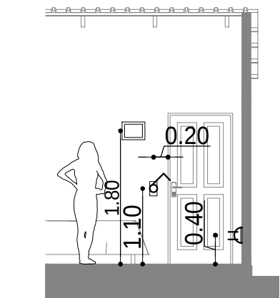
DETALLE ALTURA DE TOMACORRIENTES /INTERRUPTORES
