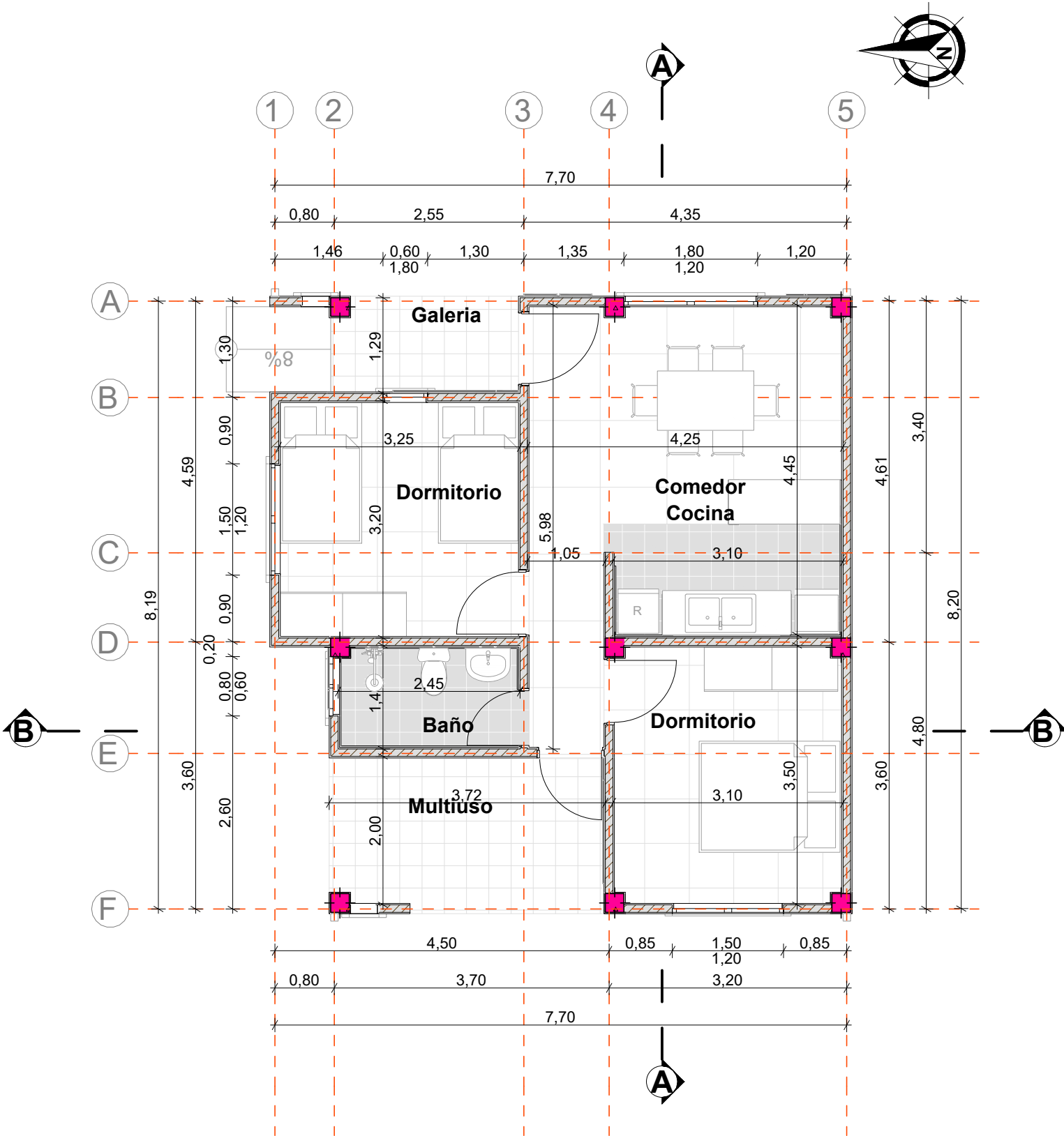
PLANTA ARQUITECTONICA
