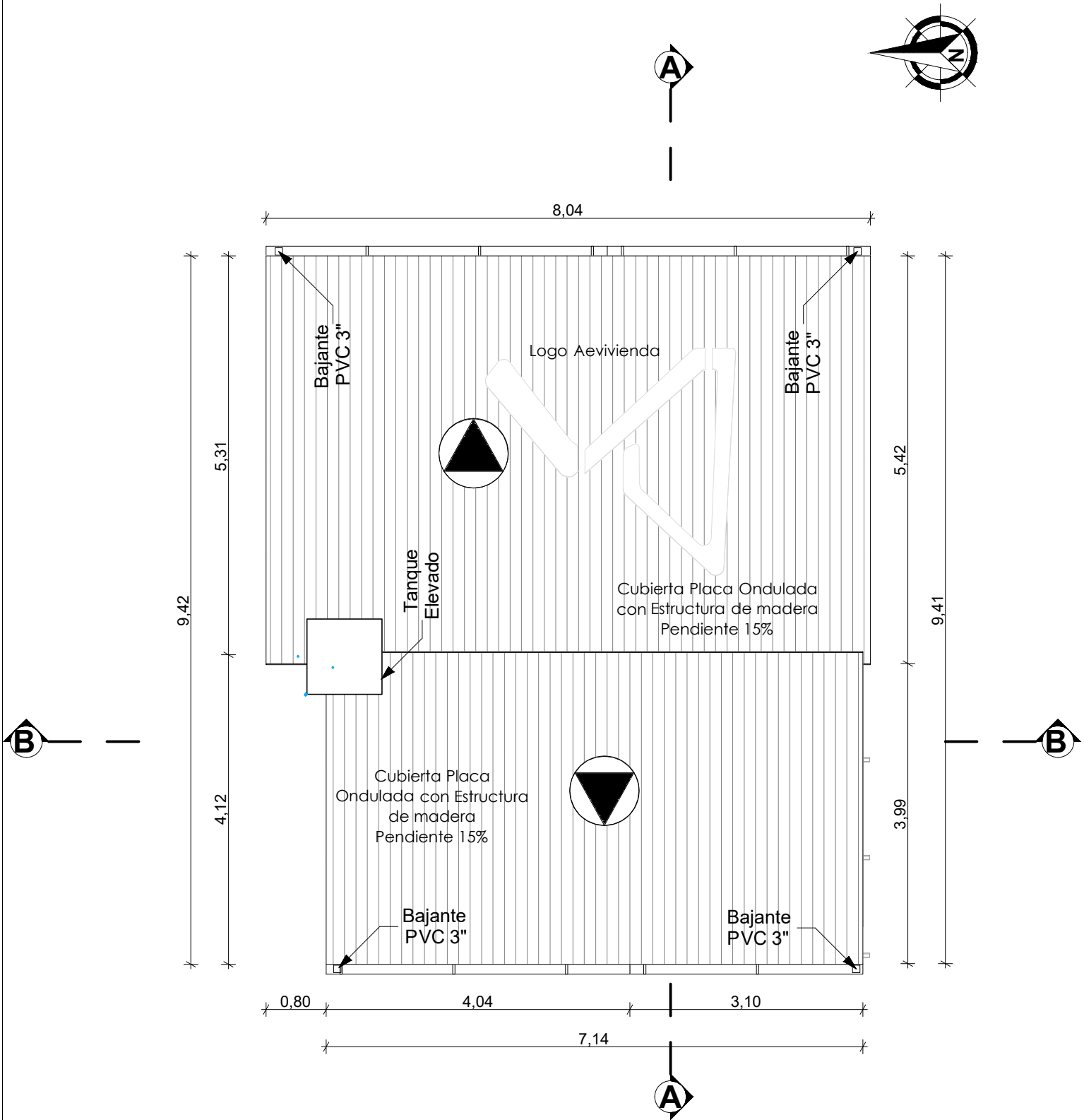
PLANO CUBIERTA
