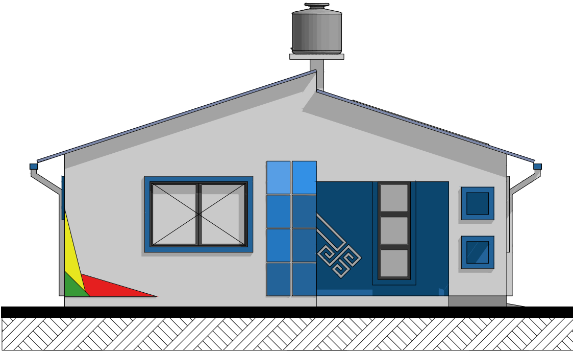
FACHADA ESTE
