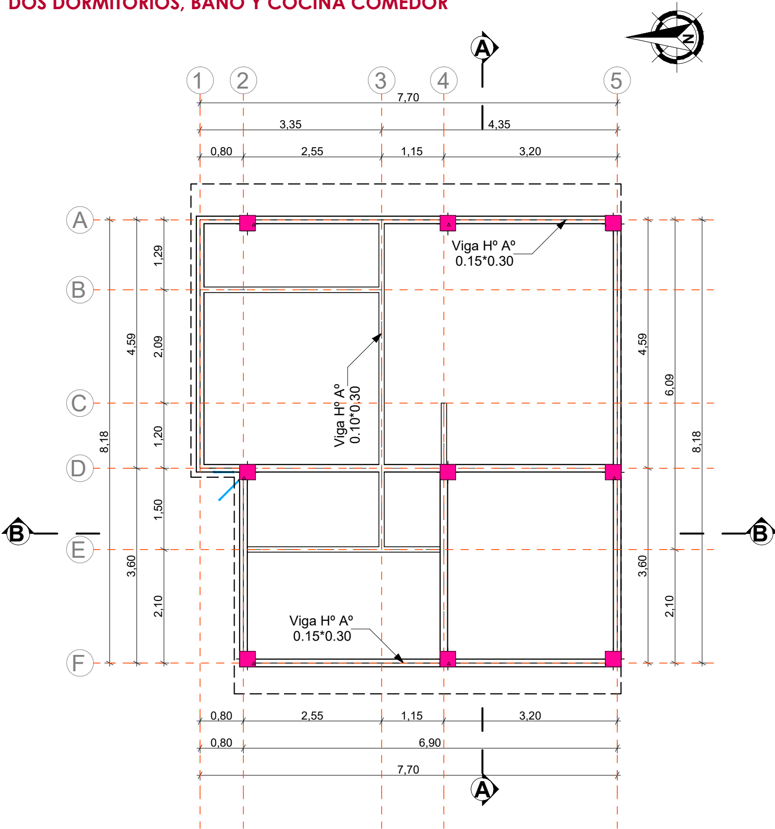
PLANO VIGA H° A°
