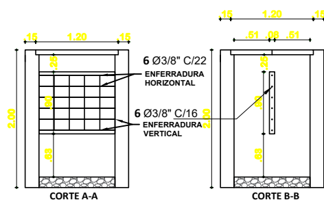
CORTE A-A
