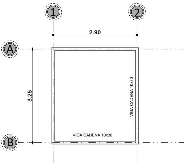
PLANO DE VIGA DE H o A o ESCALA: 1:75
