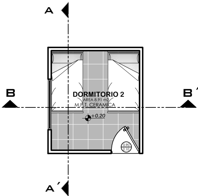
PLANTA AMOBLADA ESCALA: 1:75
