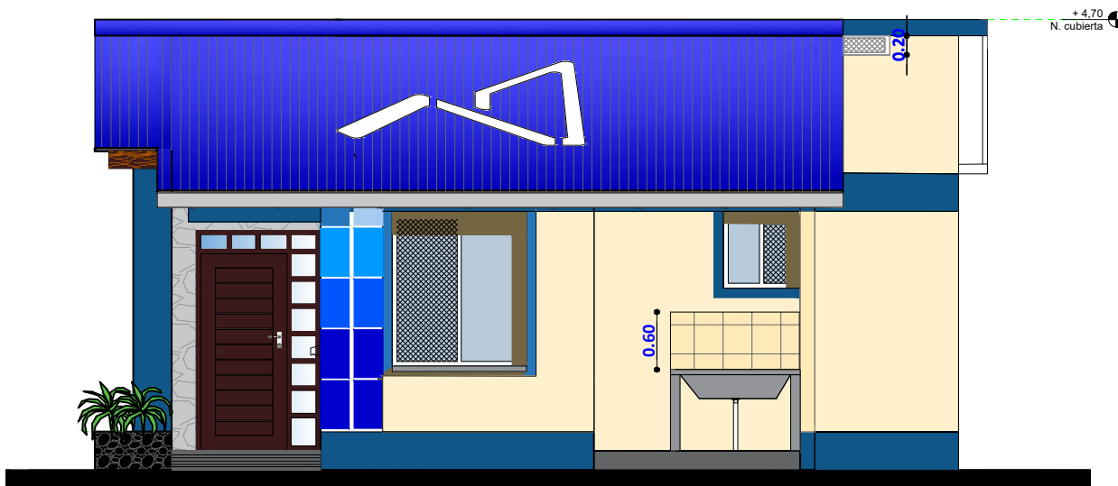
ELEVACION LATERAL DERECHA ESC. 1:75
