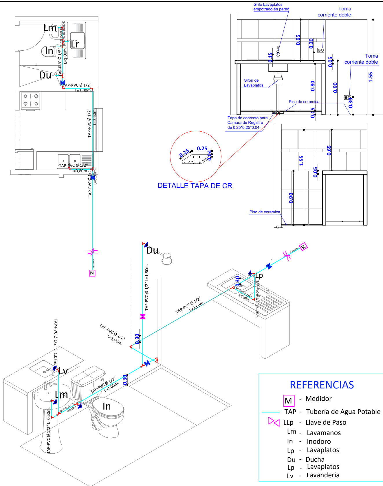
PLANO DE INSTALACION AGUA POTABLE ESC. 1:75
