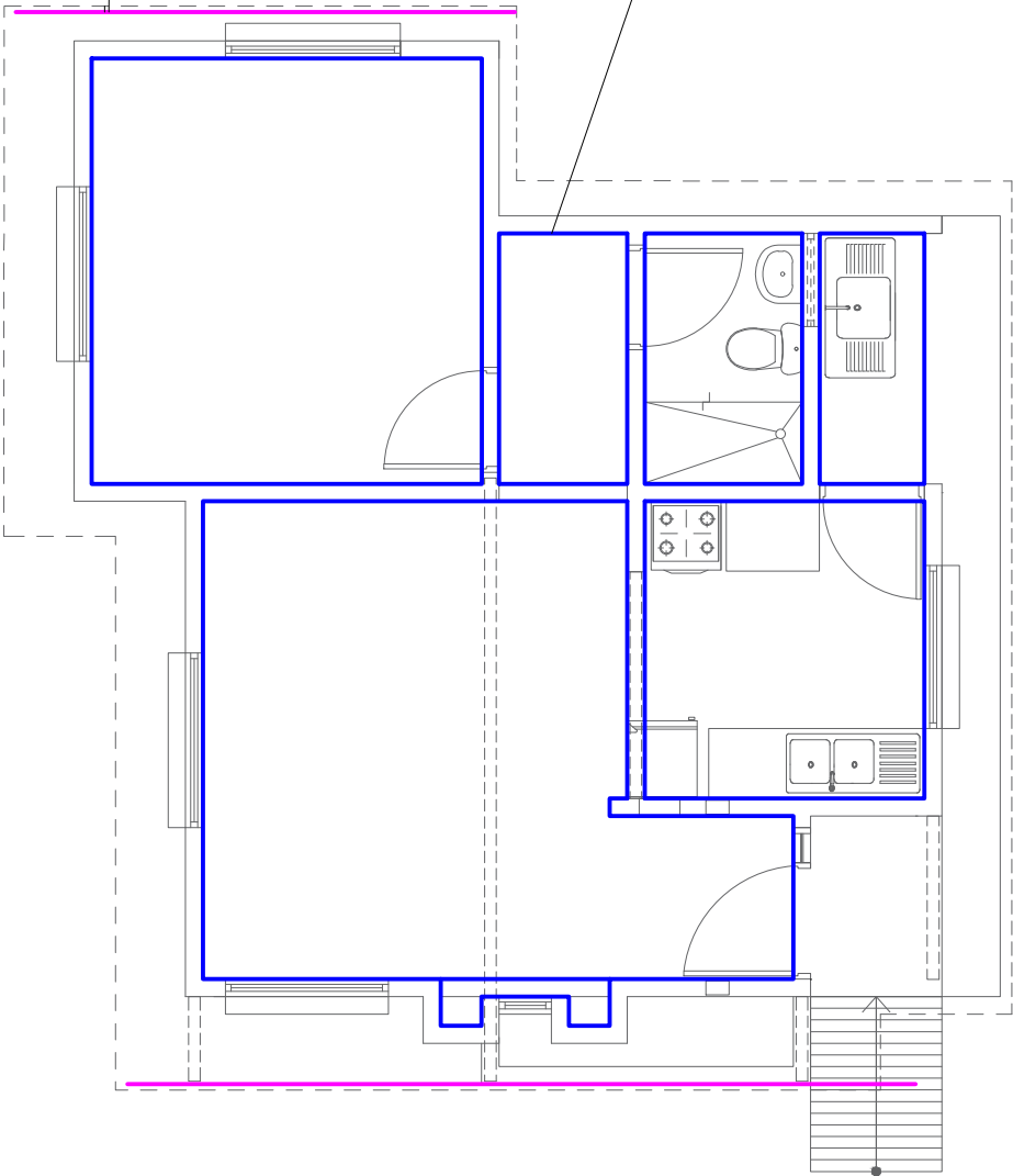
PLANO DE PVC INTERIOR - EXTERIOR ESC. 1:75
