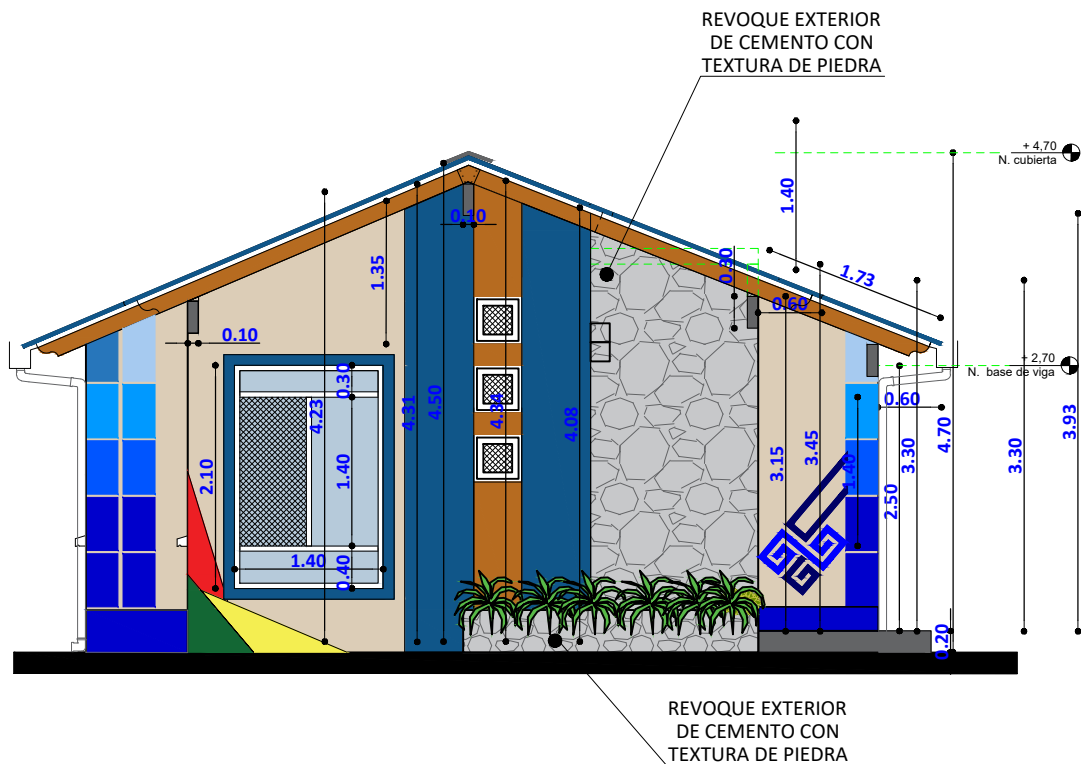
ELEVACION FRONTAL ESC. 1:75
