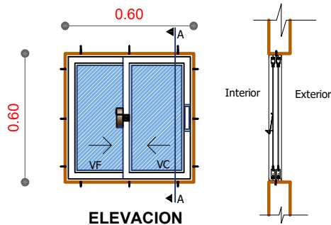
SECCION A-A
