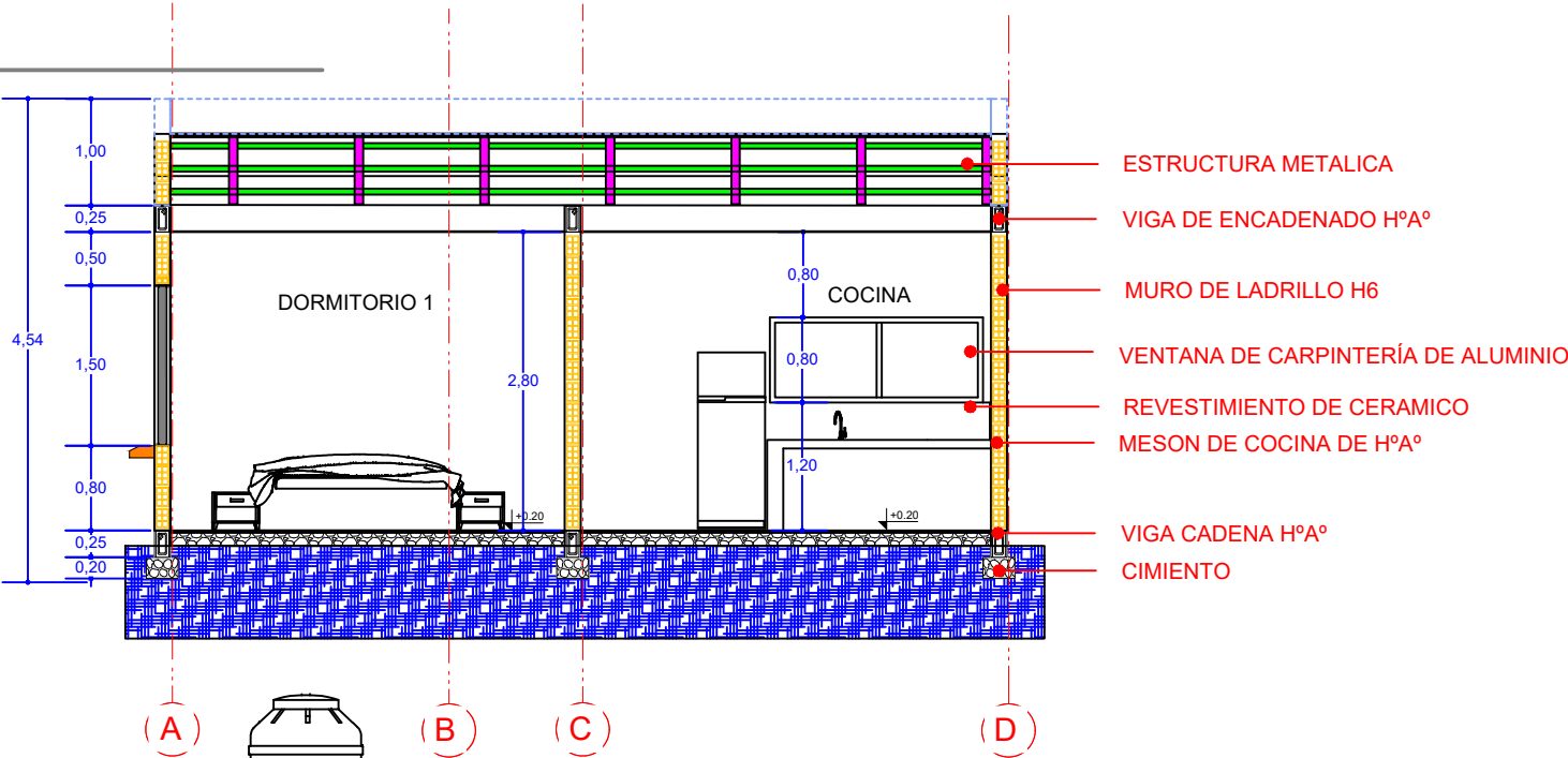
CORTE B-B
