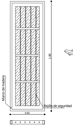
Ventana Tipo 4
