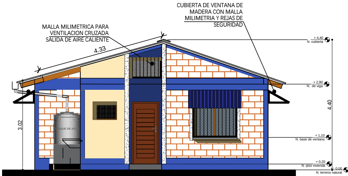
ELEVACION POSTERIOR SC. 1:75
