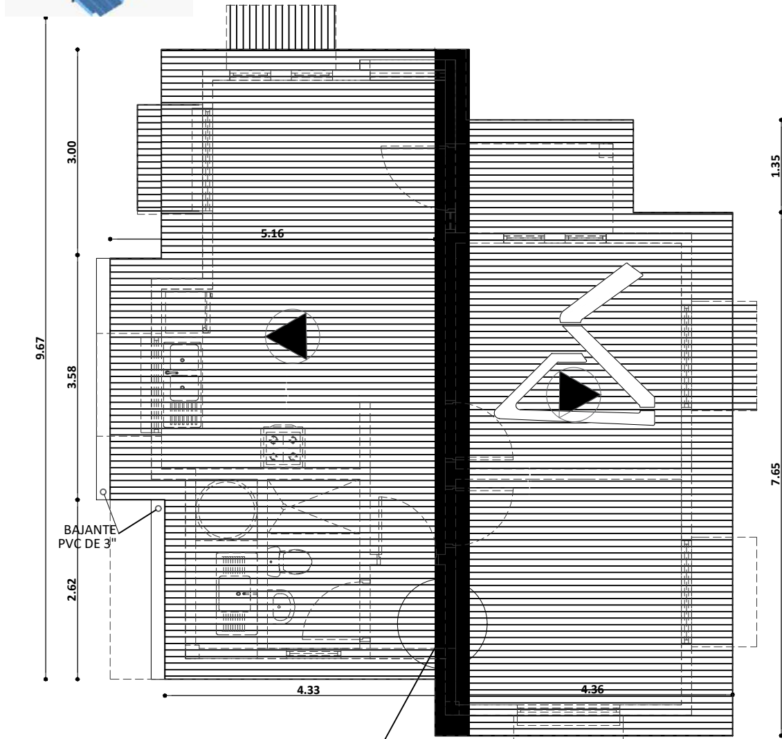
PLANO DE CUBIERTA ESC. 1:75
