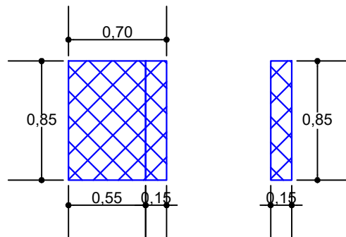
REVESTIMIENTO DE MUROS DE APOYO
