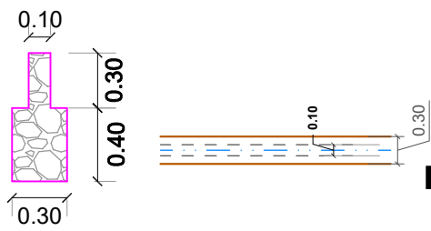
PLANTA DE SOBRECIMENTOS ESCALA: 1:75
