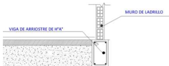
VIGA DE ARRIOSTRE DE HORMIGON ARMADO DE 0,10X0,20 M
