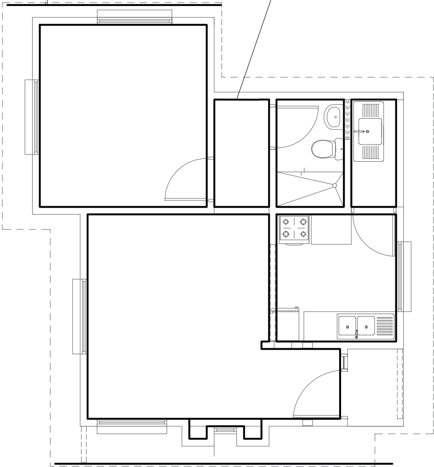
PLANO DE PVC INTERIOR - EXTERIOR ESC. 1:75
