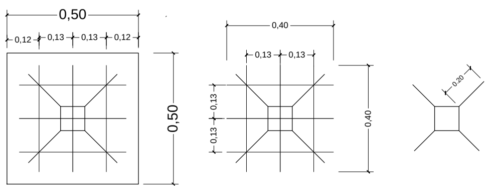
ZAPATA: DISPOSICION DE FIERROS DE 12 mm - 1/2 EN DOS DIRECCIONES
