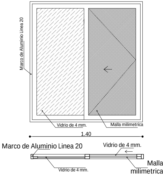
Ventana Tipo 2
