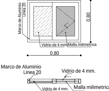
Ventana Tipo 3
