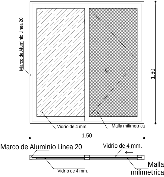
Ventana Tipo 1
