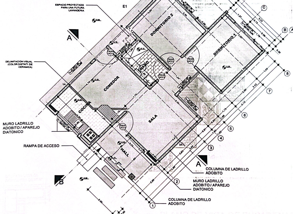
3 PLANTA TECNICA ACOTADA Scale: 1:100
