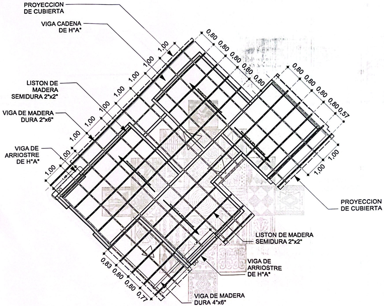
5 PLANO DE ESTRUCTURA DE MADERA PARA CUBIERTA Scale: 1:100
