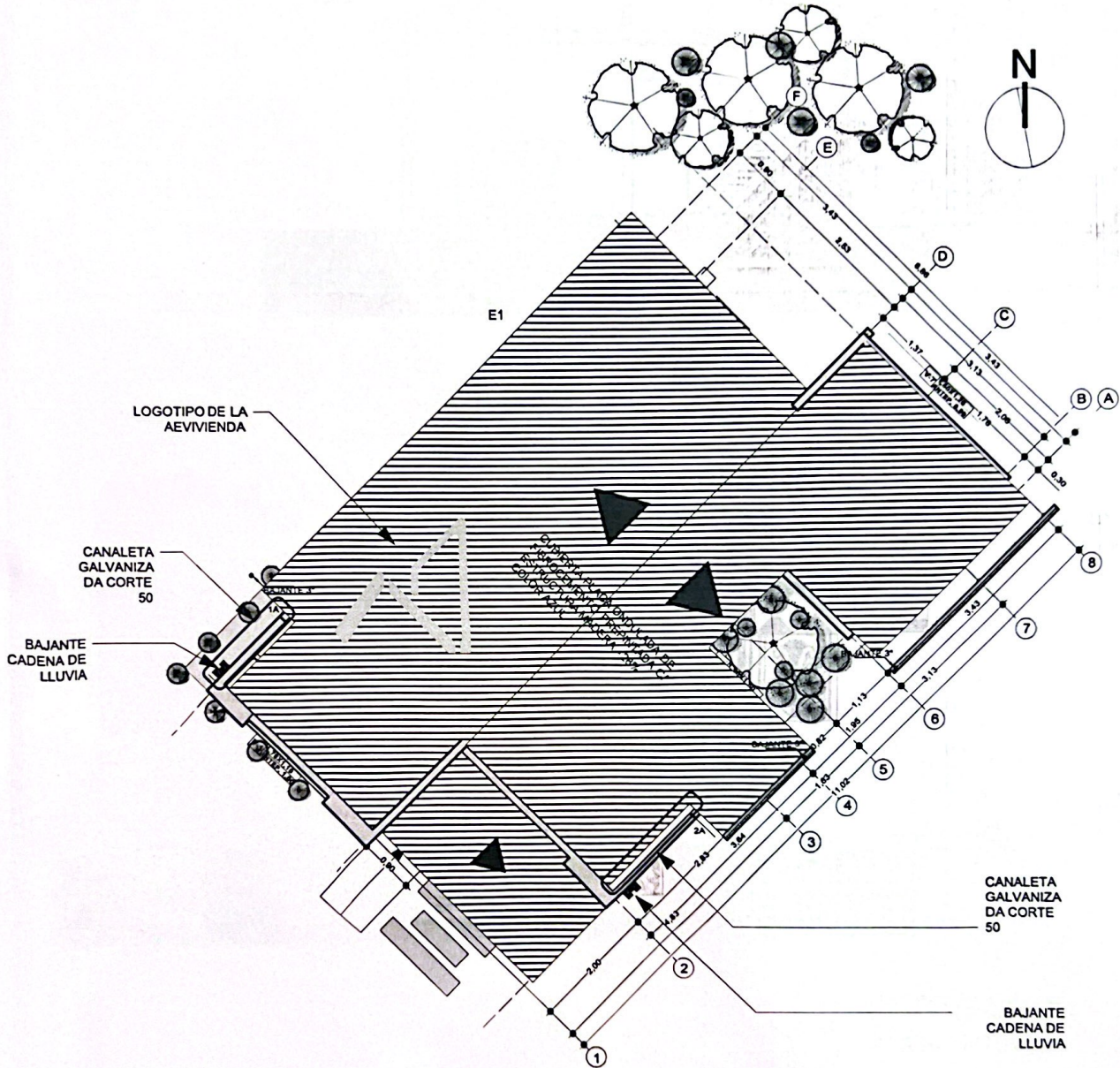
7 PLANO DE CUBIERTA Scale: 1:100
