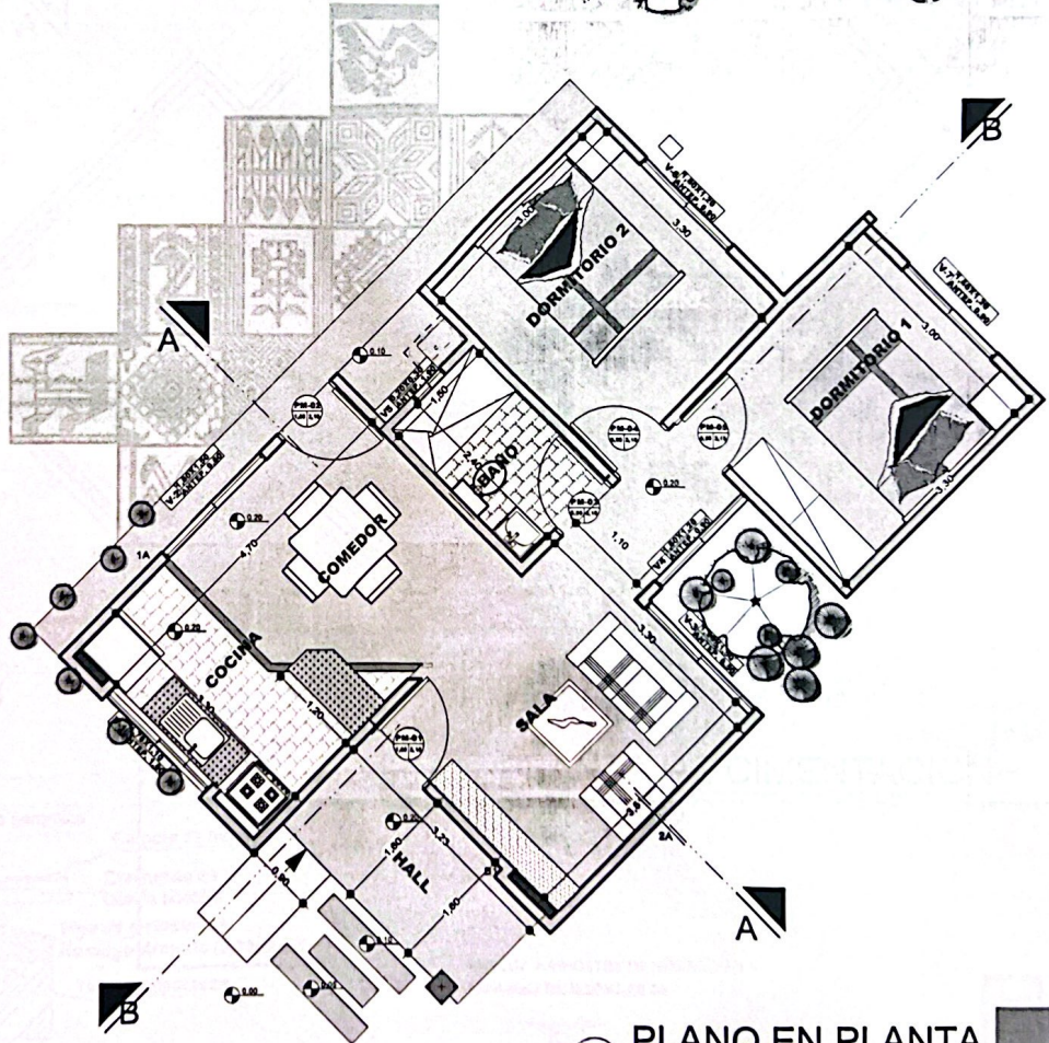
1 PLANO EN PLANTA Scale: 1:100
