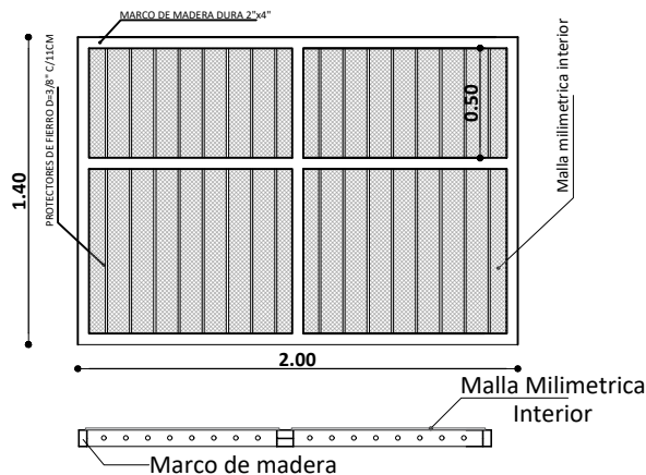
Ventana Tipo 2
