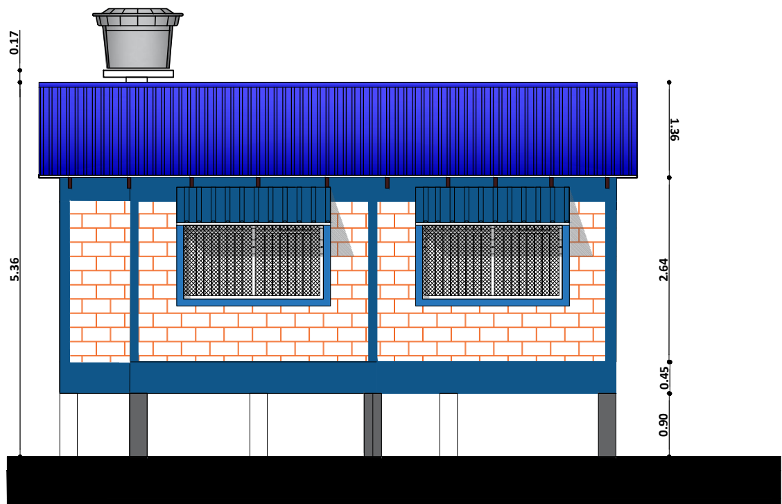
ELEVACION LATERAL IZQUIERDO ESC. 1:75
