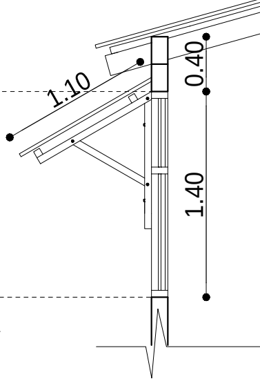
DETALLE DE CUBIERTA SOBRE VENTANA
