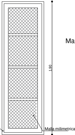
Ventana Tipo 4
