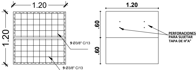
PLANTA
