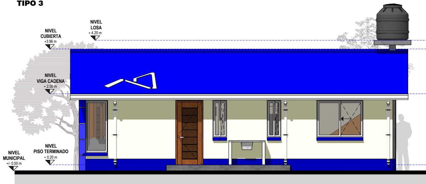
TIPO 3 POSTERIOR ESC. 1:75
