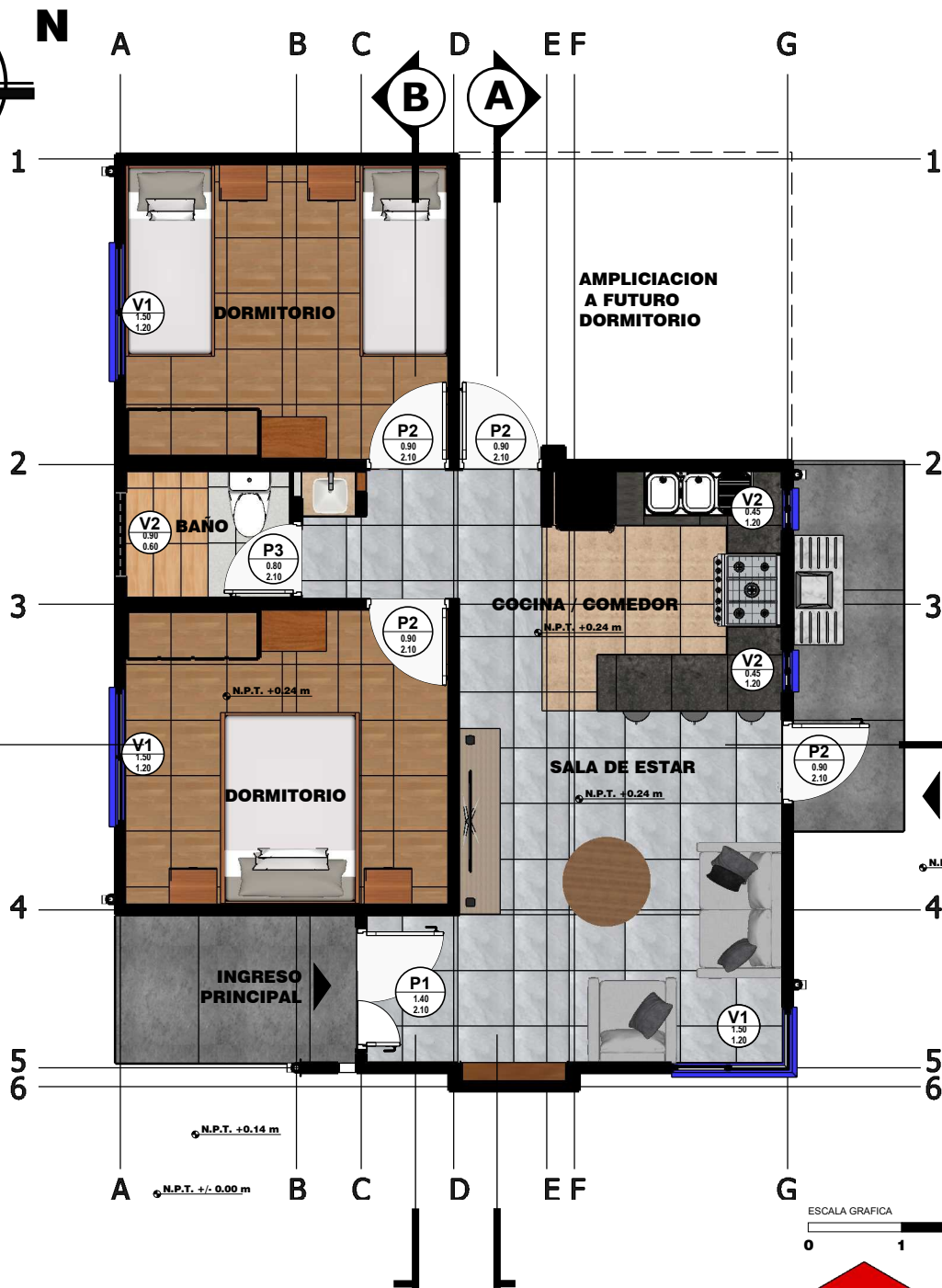
PLANTA ESC. 1:75
