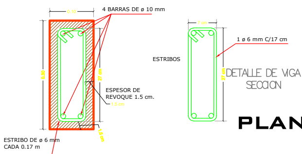
DETALLE DE VIGA 0.10 x 0.30
