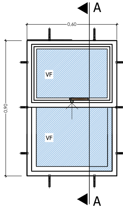
ELEVACION
