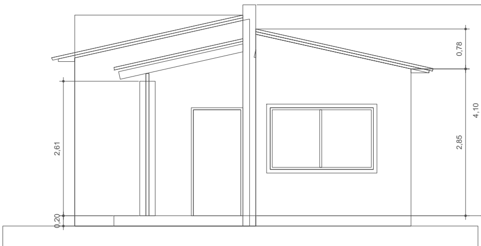
10 FACHADAS Scale: 1:75
