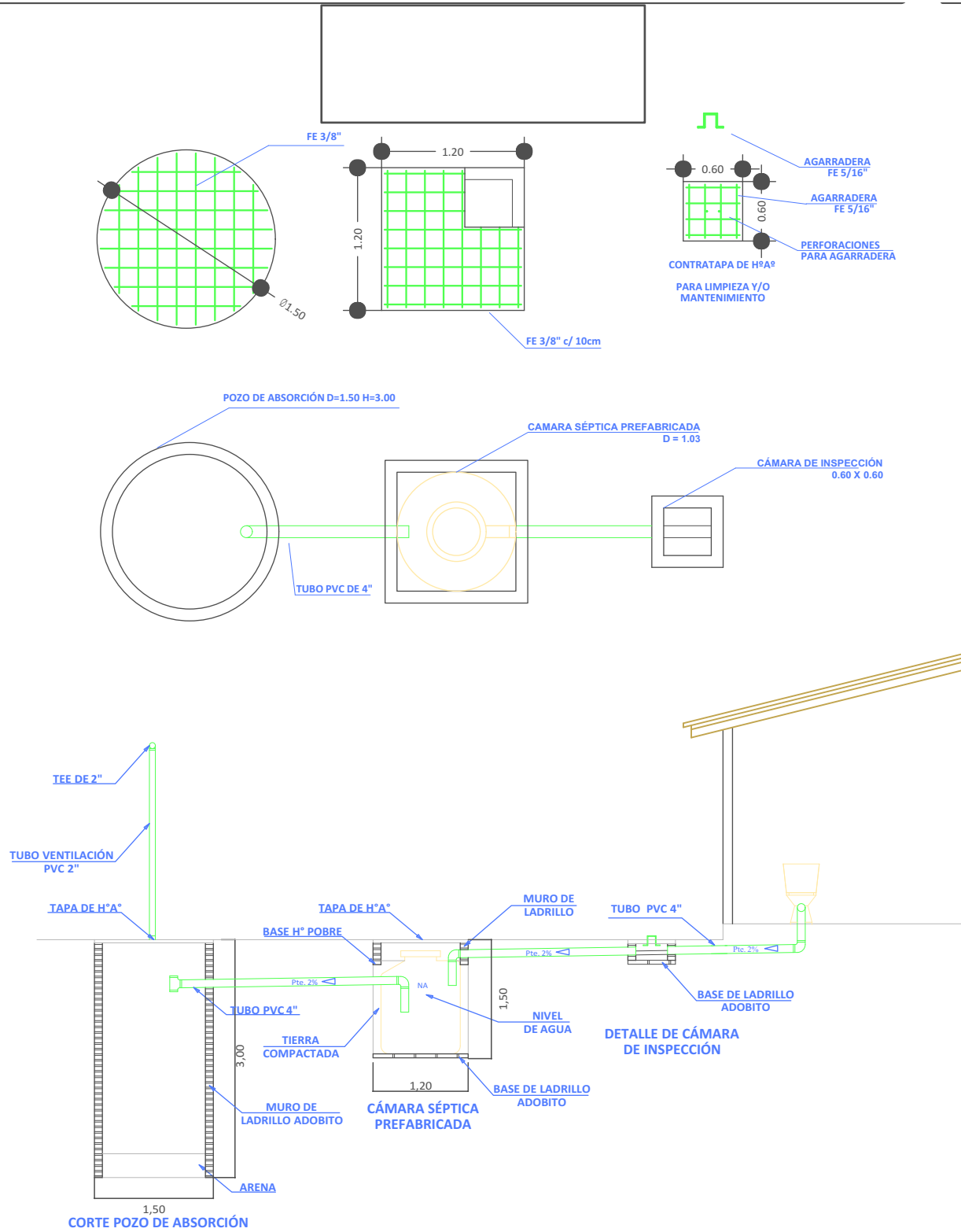
19 SISTEMA DE DESCARGA SANITARIO Scale: 1:75
