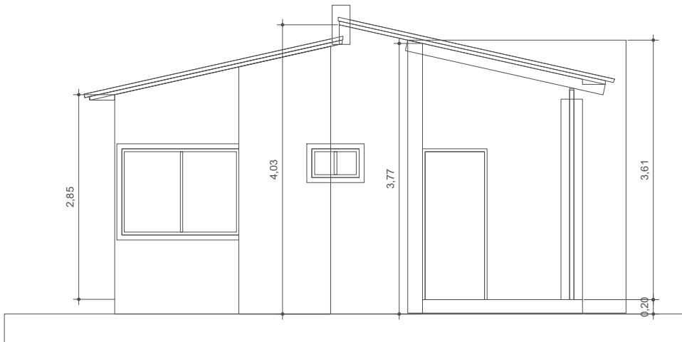
10 FACHADAS Scale: 1:75
