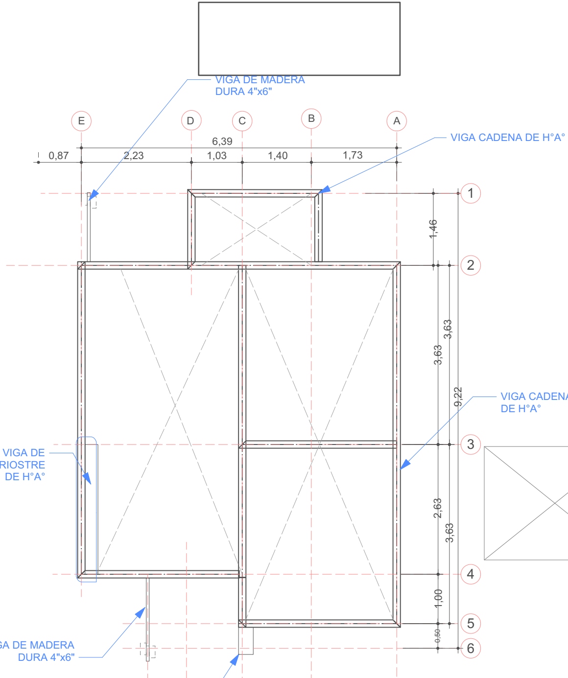
4 PLANO DE VIGA ENCADENADO Scale: 1:75
