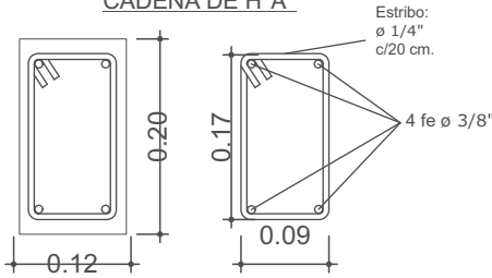
DETALLE VIGA DE H°A°
