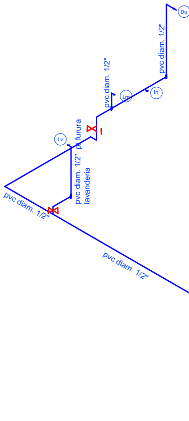
16 PLANO ESQUEMATICO ISOMETRICO - DE INSTALACION HIDRAULICA Scale: 1:100
