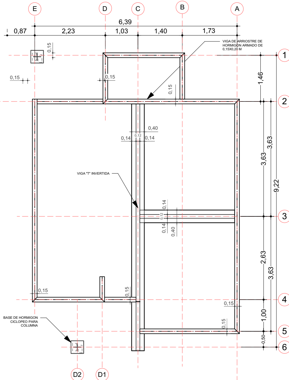
1 PLANO DE CIMENTACION
