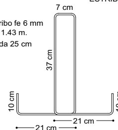
SECCION VIGA T
