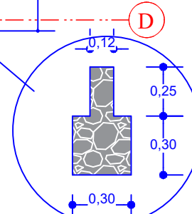
DETALLE DE CIMENTO MURO BAÑO C 2-3
