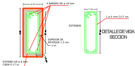
DETALLE DE VIGA 0.10 x 0.30
