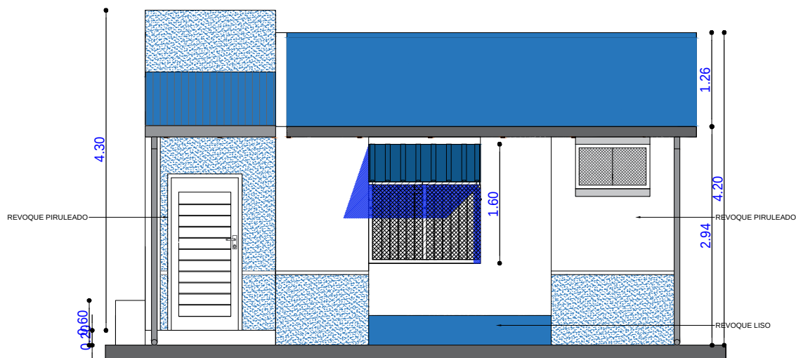
ELEVACION LATERAL ESC. 1:75
