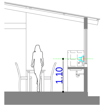
DETALLE ALTURA DE TOMACORRIENTES
