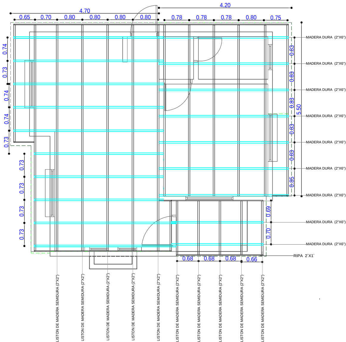
PLANO DE VIGAS EN CUBIERTA ESC. 1:75
