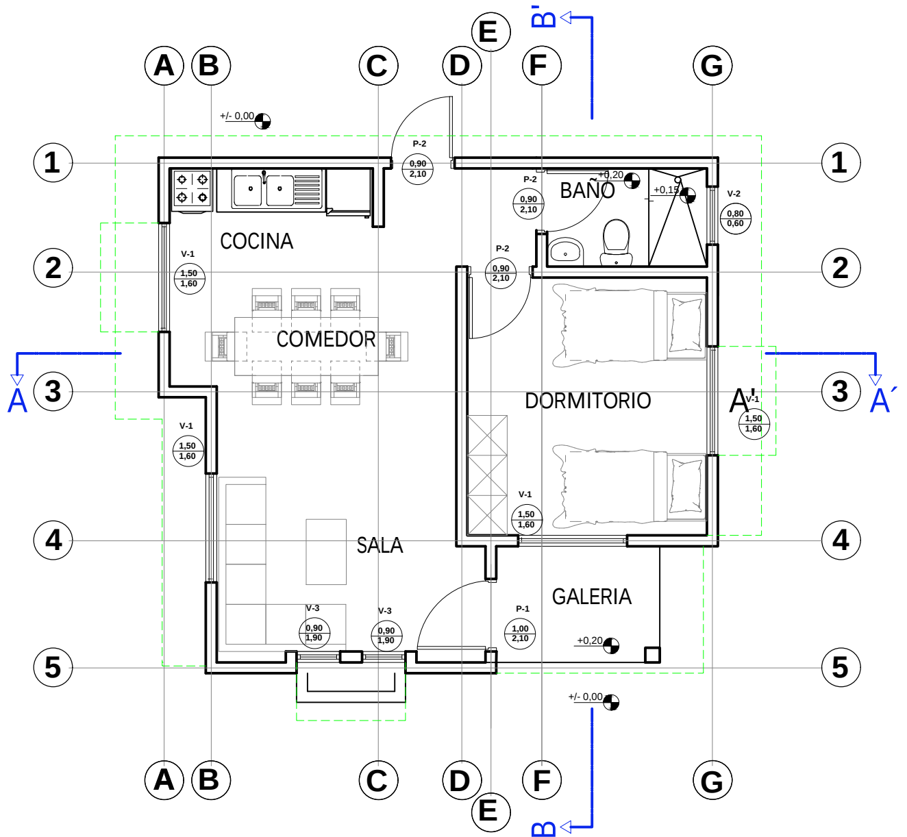
PLANTA AMOBLADA ESC. 1:75
