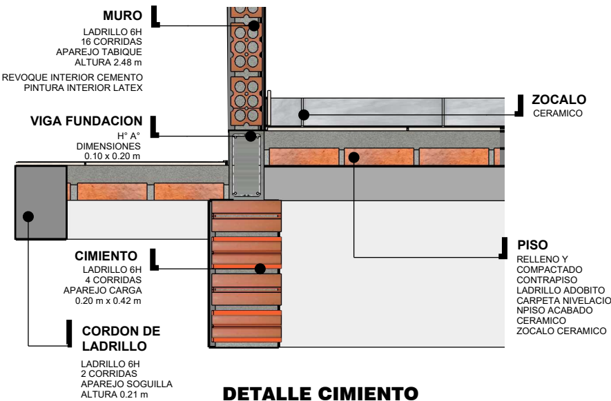
DETALLE CIMIENTO ESC. 1:15
