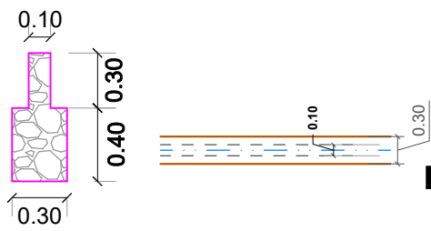
PLANTA DE SOBRECIMIENTOS ESCALA: 1:75
