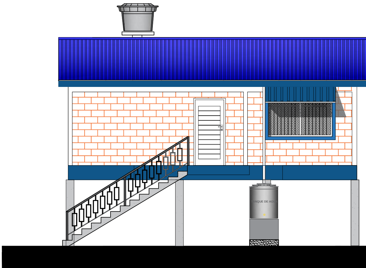
ALZADO SUR ESC. 1:75
