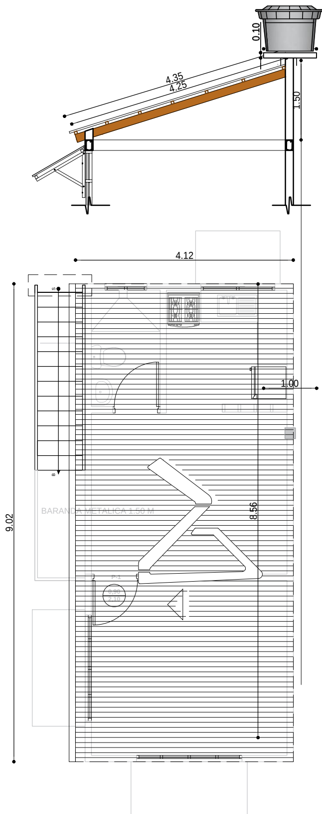
PLANO DE CUBIERTA ESC. 1:75
