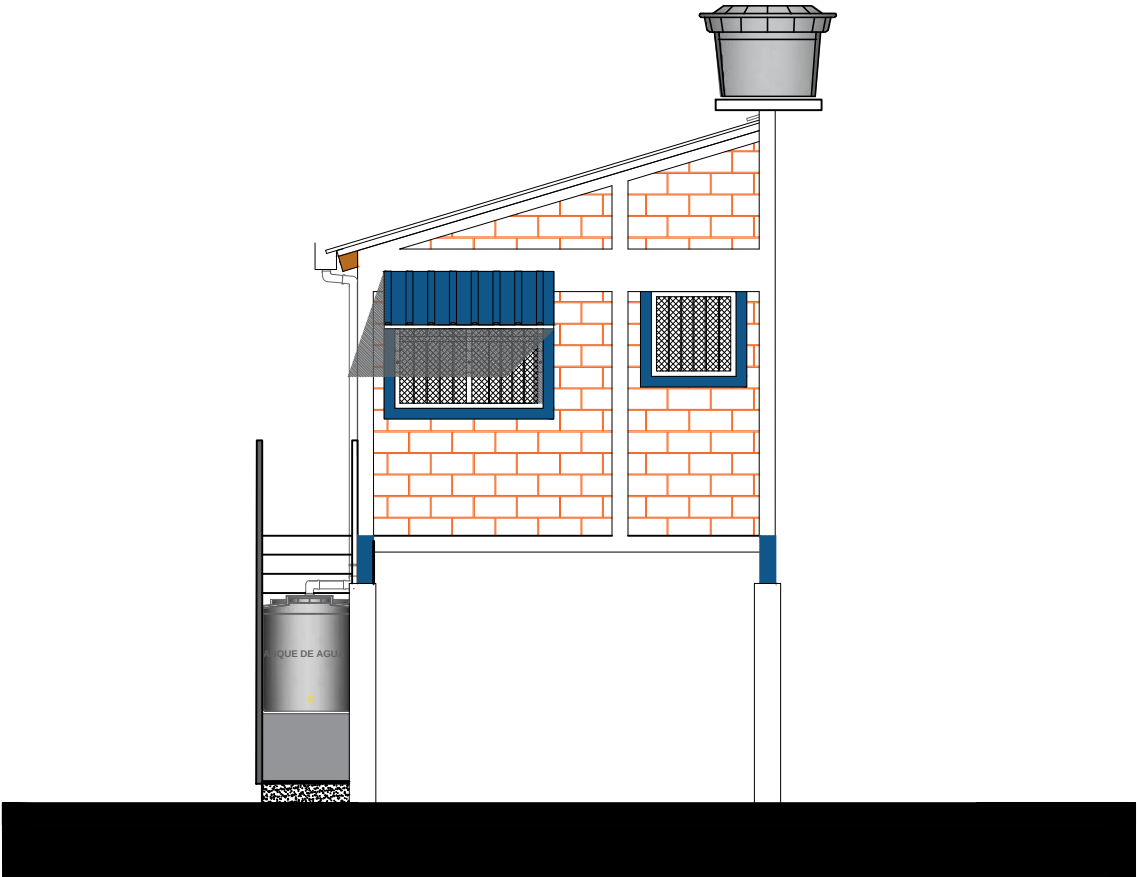
ALZADO ESTE ESC. 1:75
