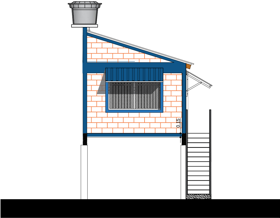
ALZADO OESTE ESC. 1:75
