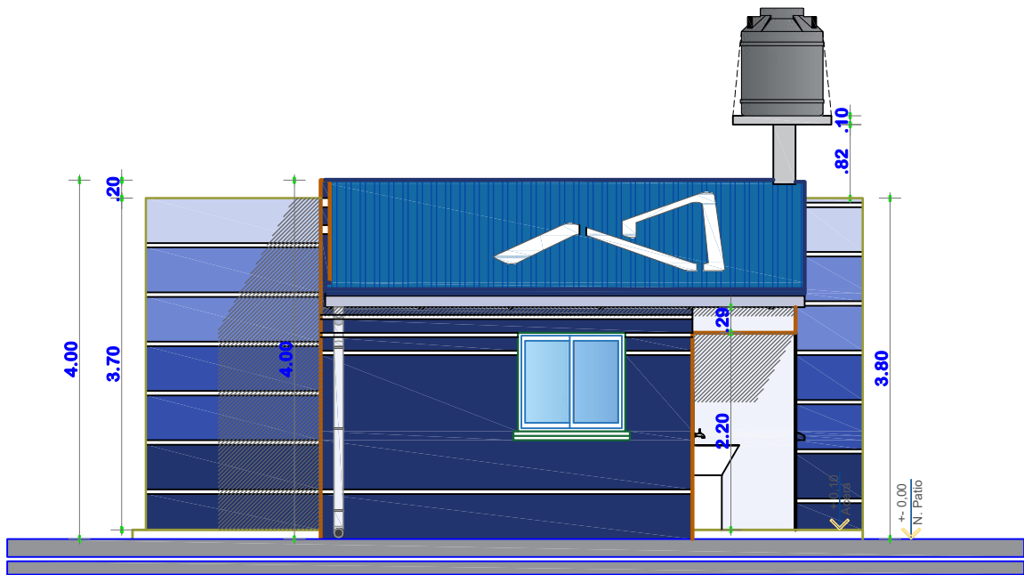
ELEVACION LATERAL DERECHO ESCALA: 1:75
