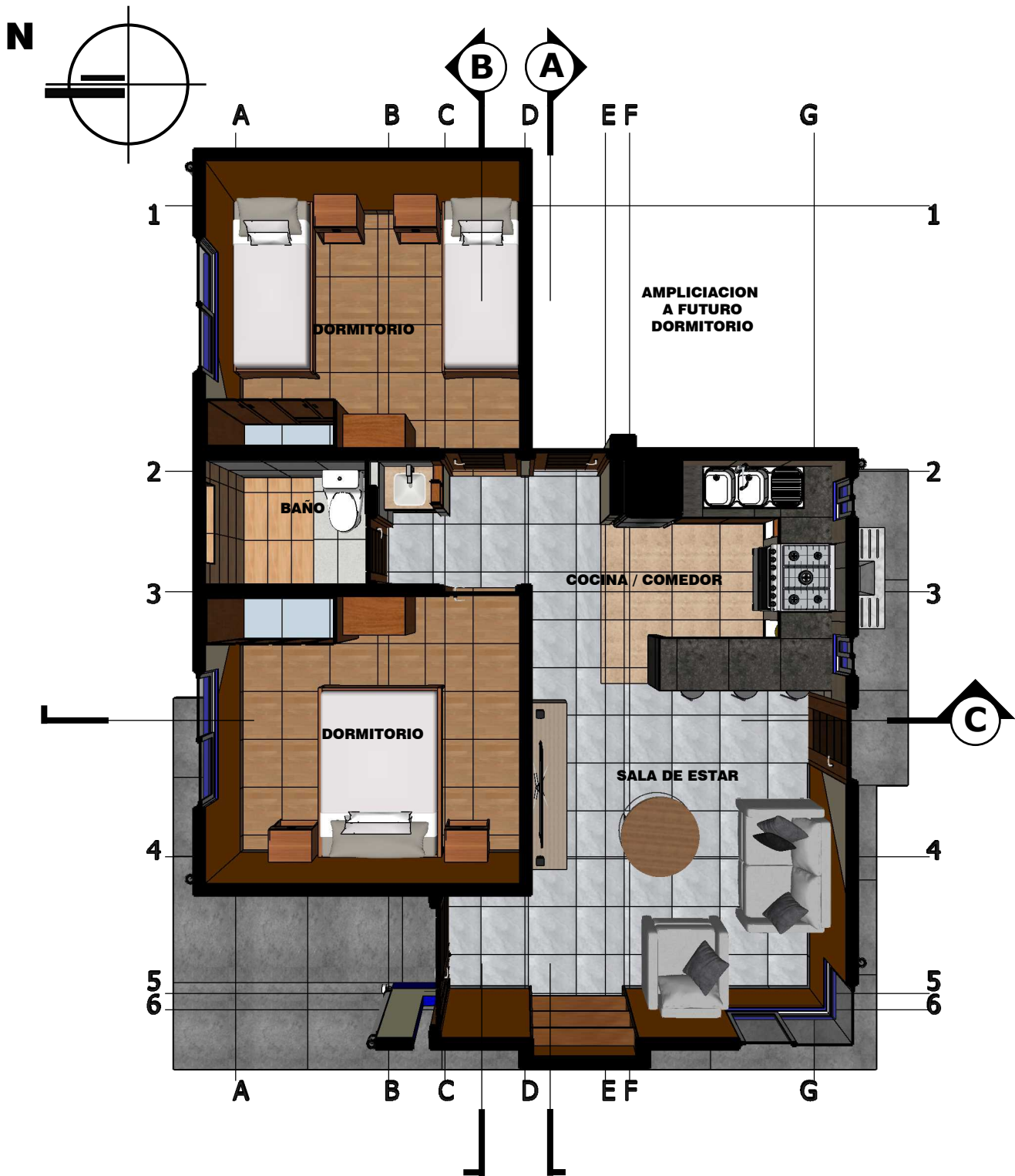
PLANTA FUGADA ESC. 1:75
