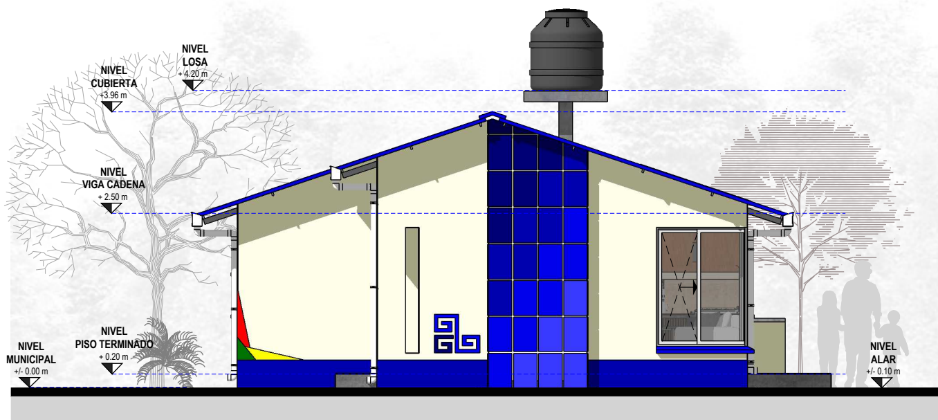
TIPO 1 FRONTAL ESC. 1:75
