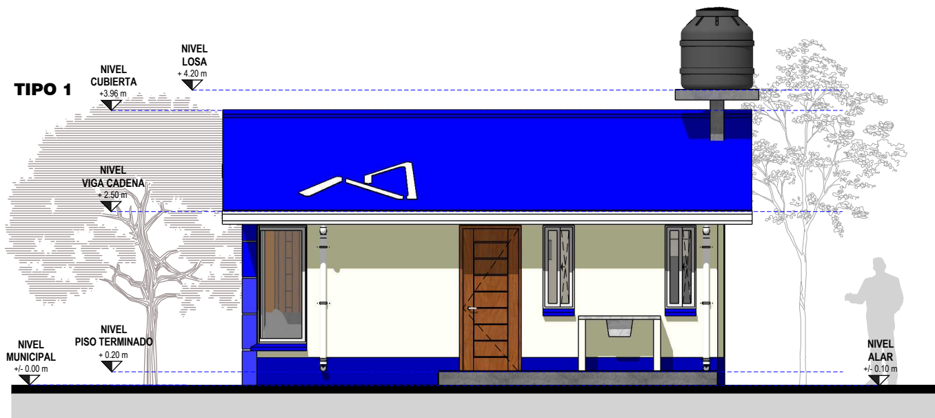
TIPO 1 POSTERIOR ESC. 1:75
