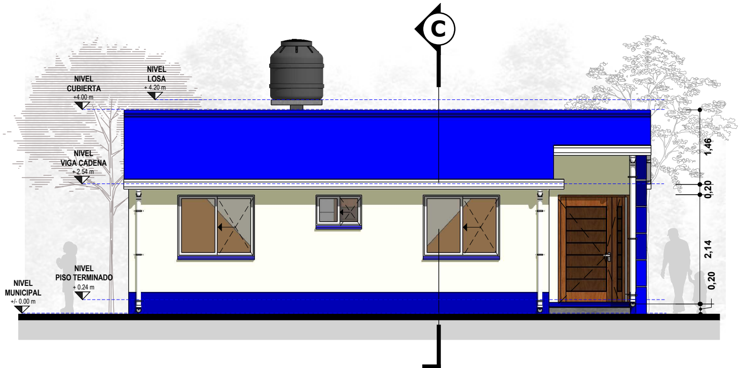
LATERAL ESC. 1:75
