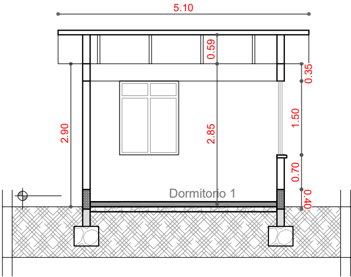
CORTE B - B''
