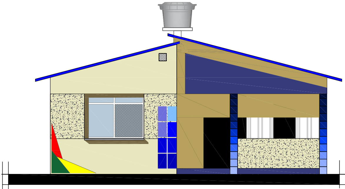
ELEVACION LATERAL 1
