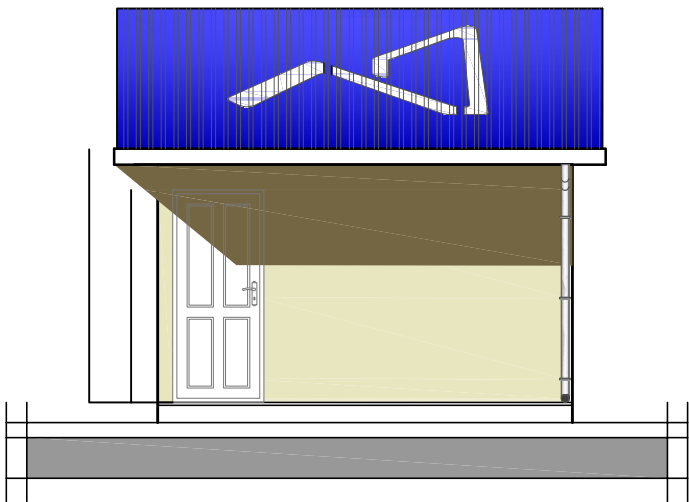
ELEVACION PRINCIPAL
