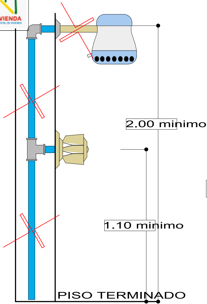
DETALLE DE DUCHA ESCALA: 1:20
