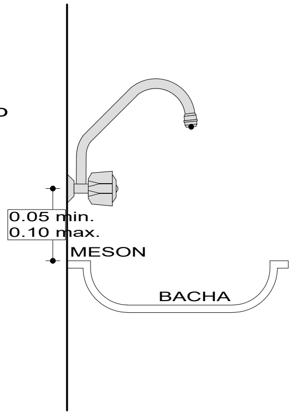
DETALLE DE GRIFO ESCALA: 1:20
